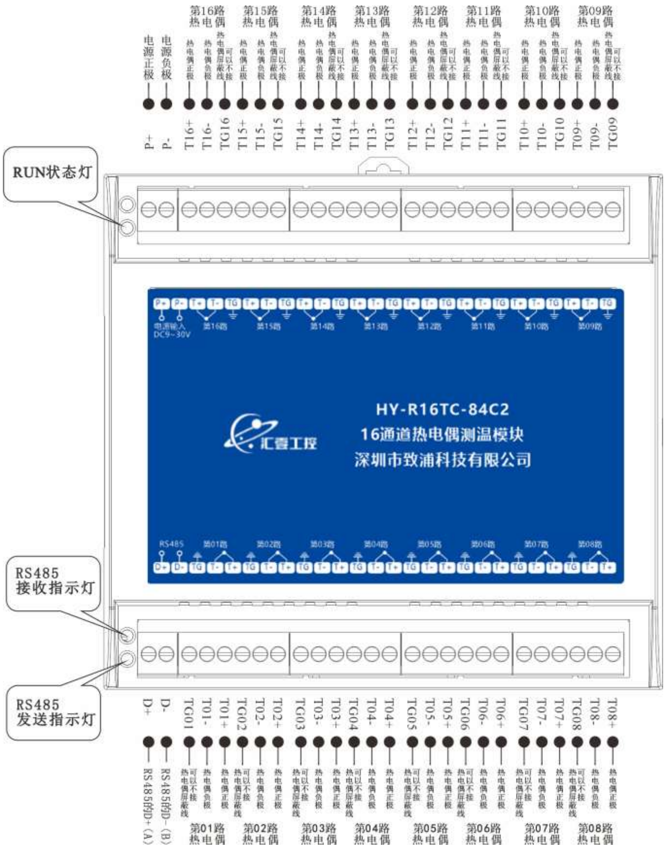
图 5.2.1: RS485 接口版本接线图
