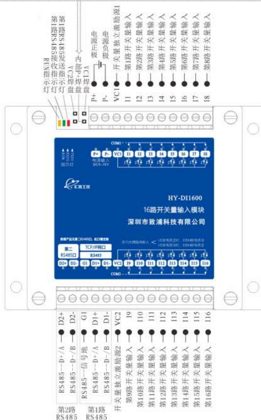
图 6.1 RS485 接口型端口定义参考图
