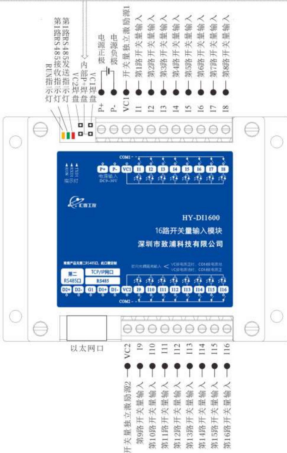
图 6.2 TCP/IP 网口接口型端口定义参考图
