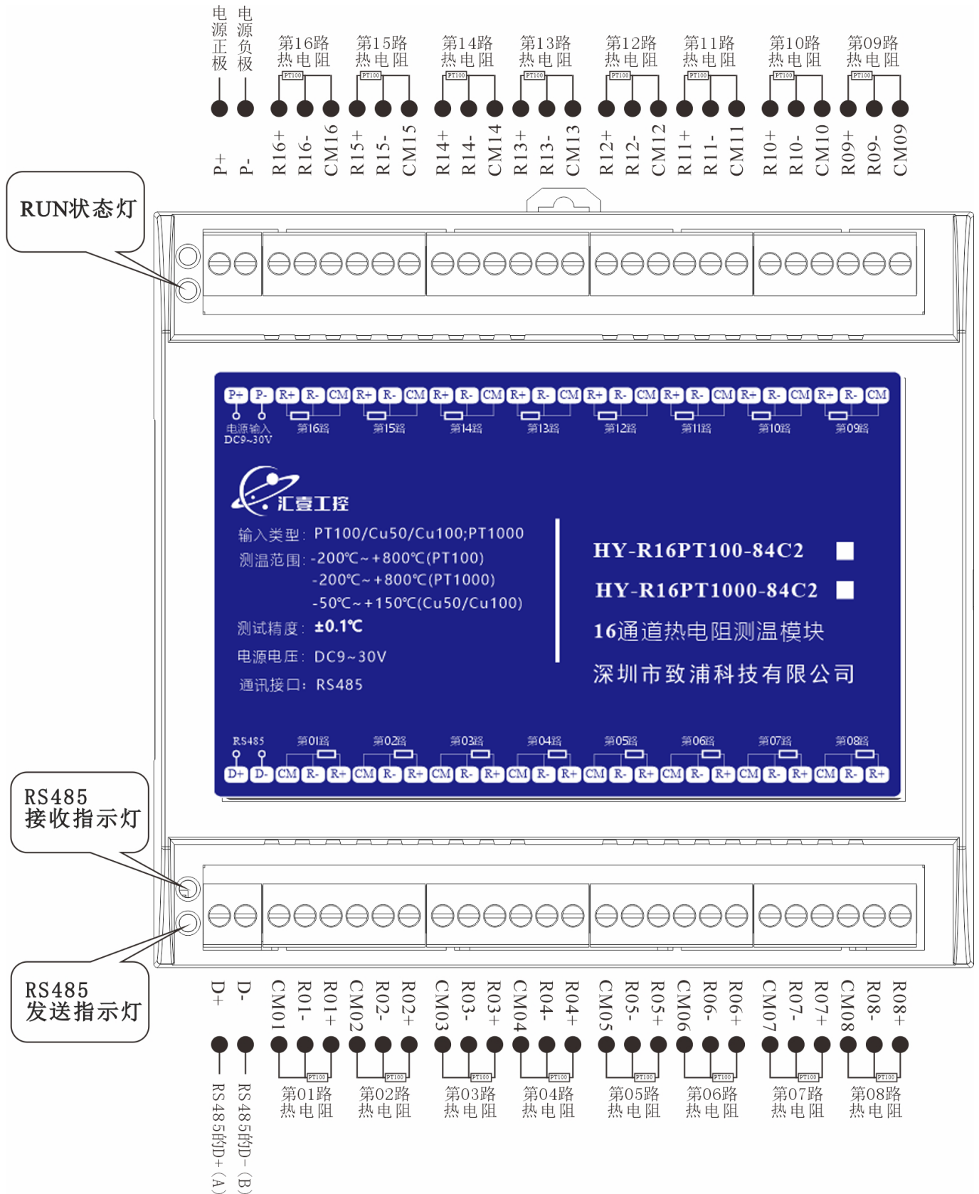
图 5.2.1：RS485 接口版本接线图
